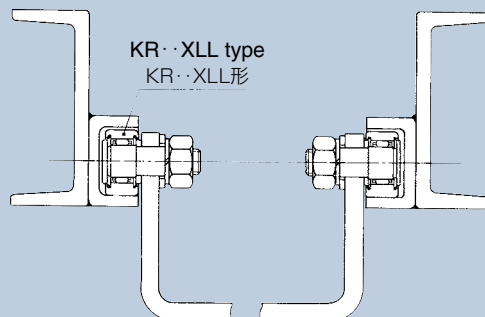
Circular conveyor supporting roller 円形コンベヤの支持ローラ
